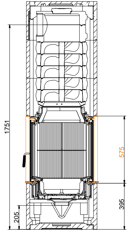
SCHNITT A-A
