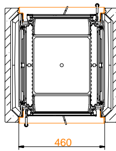
SCHNITT B-B
