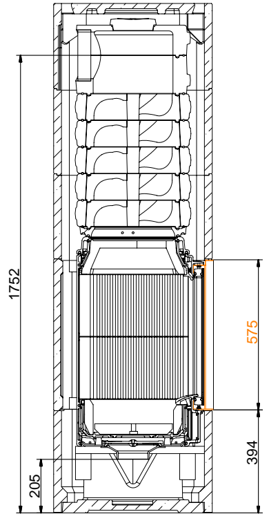
SCHNITT A-A
