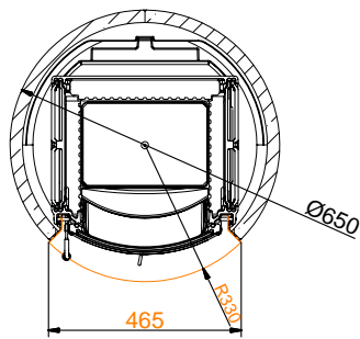
SCHNITT B-B
