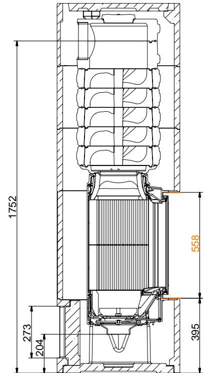
SCHNITT A-A
